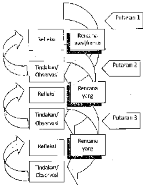
Gambar 3.1 Alur PTK
